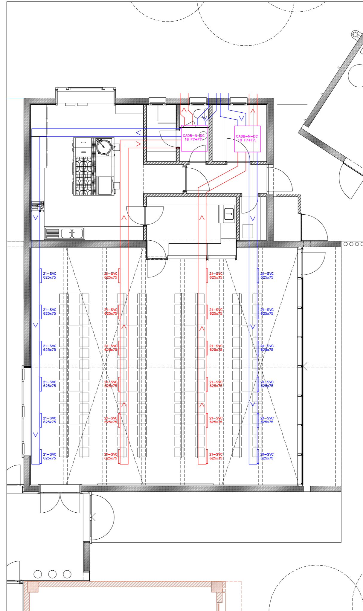
INSTALACIÓN CLIMATIZACIÓN. VENTILACIÓN. ESCALA: 1:100
