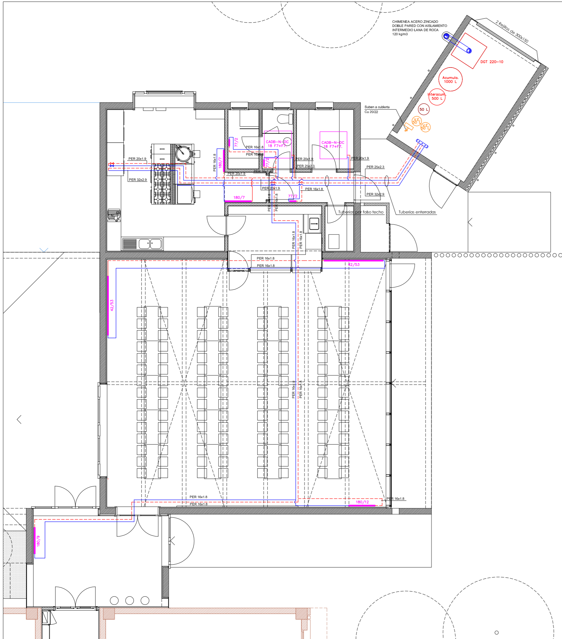
INSTALACIÓN CLIMATIZACIÓN. RADIADORES. ESCALA: 1:100
