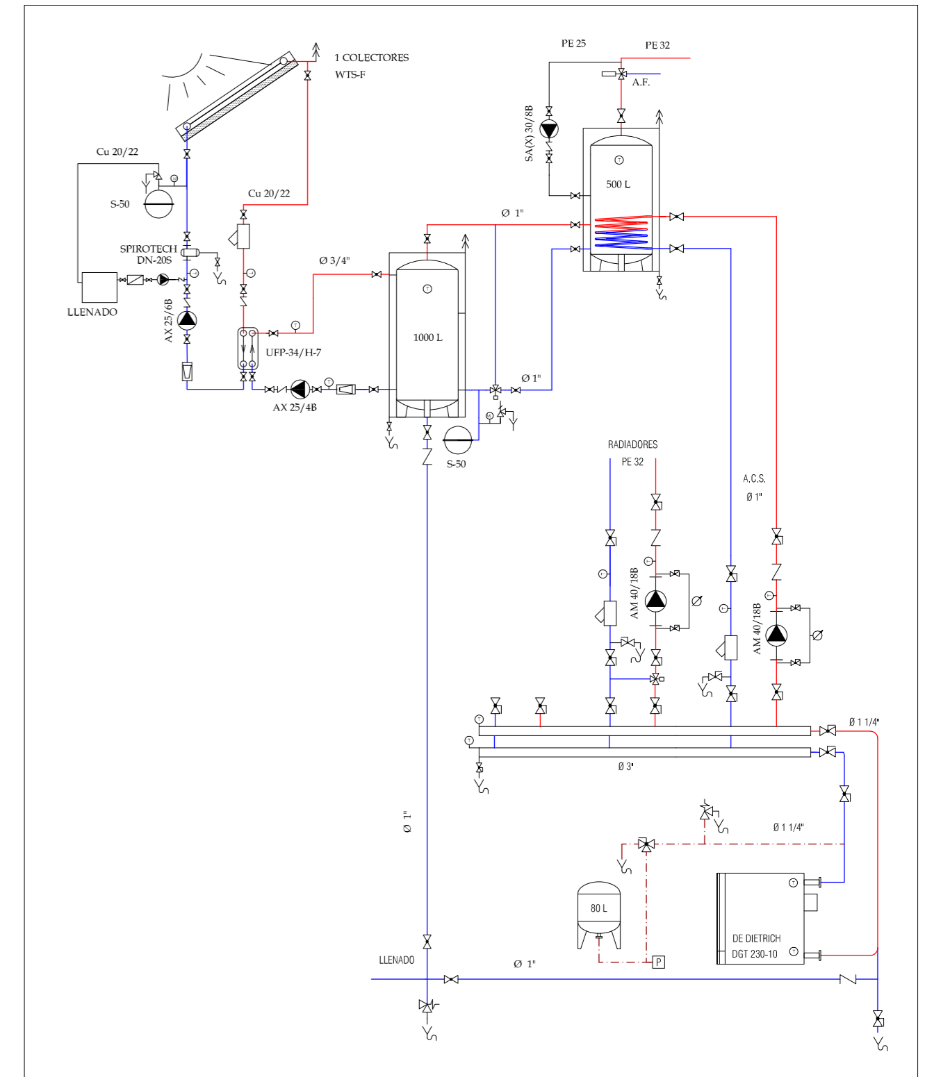
ESQUEMA DE PRINCIPIO
