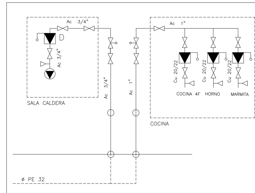
LÍNEA GAS NATURAL
