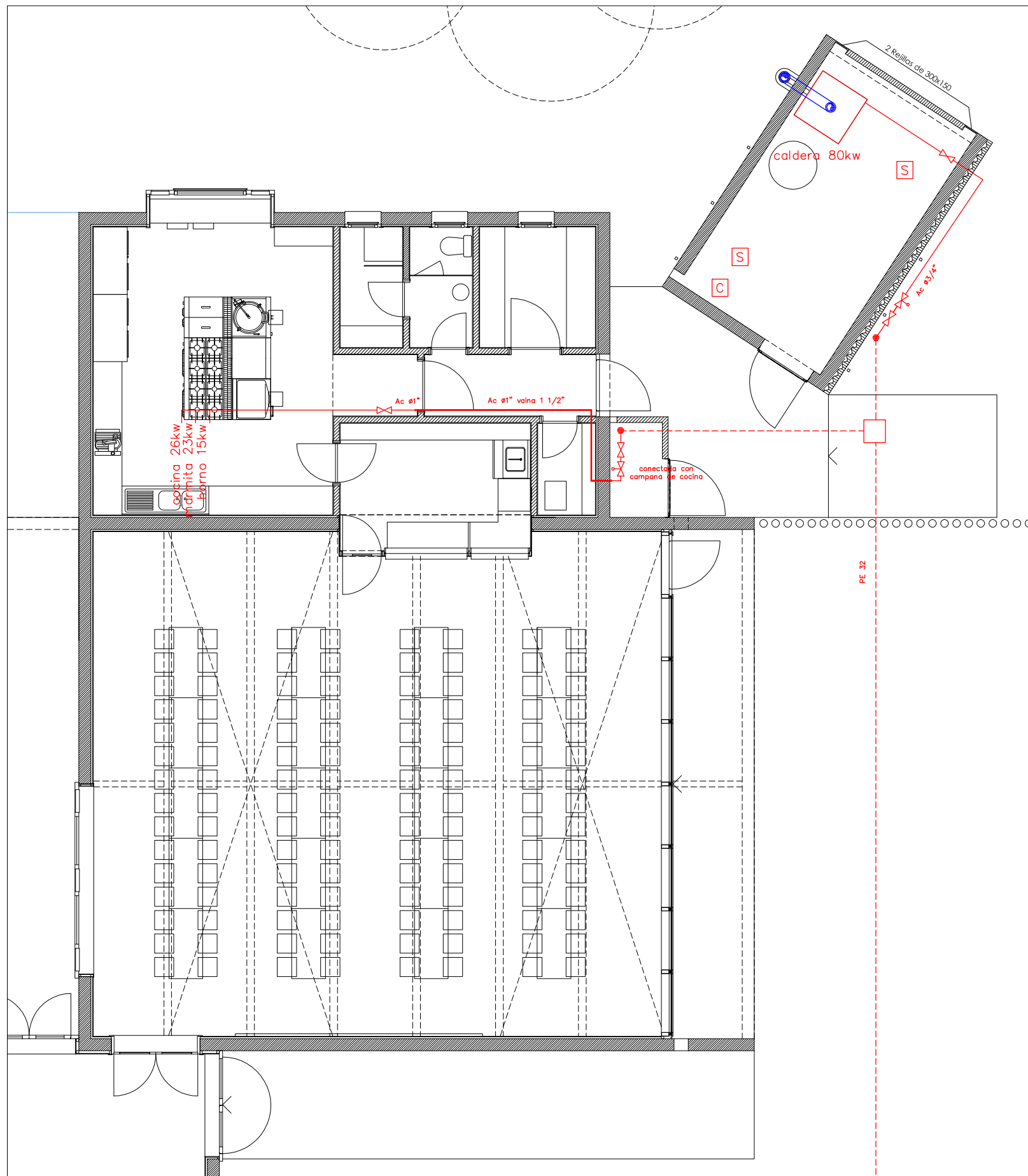
INSTALACIÓN DE GAS.
