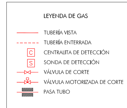
LÍNEA GAS NATURAL
