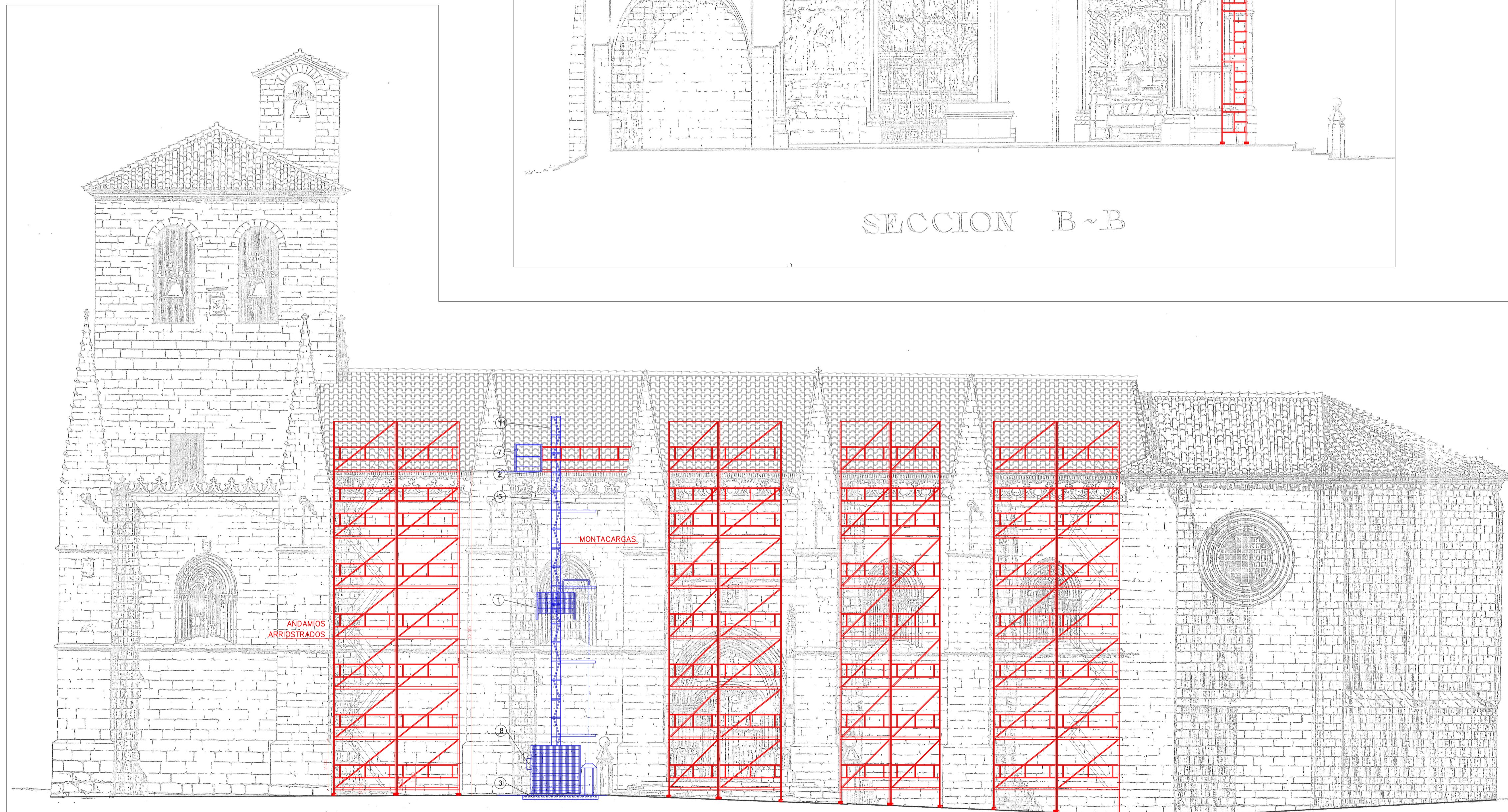
ALZADO SVR
