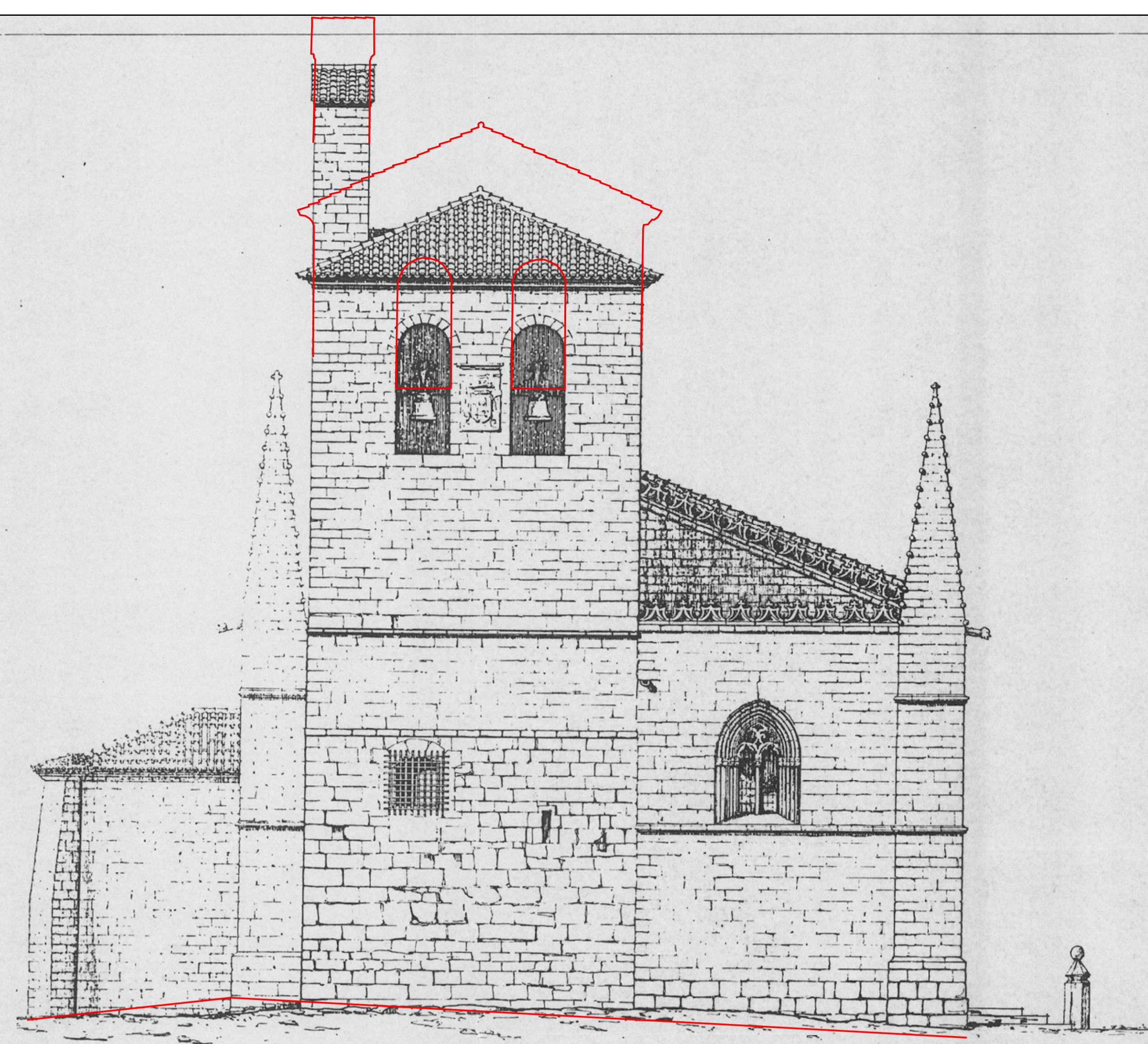
ALZADO OESTE
