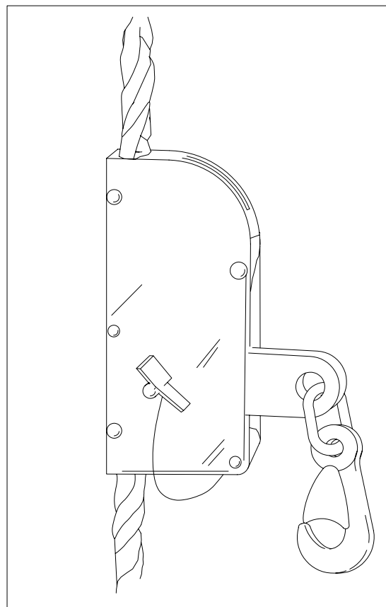
Anclaje móvil para cinturón de seguridad
