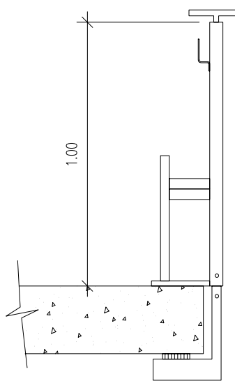
SOPORTE " TIPO - 3 "
