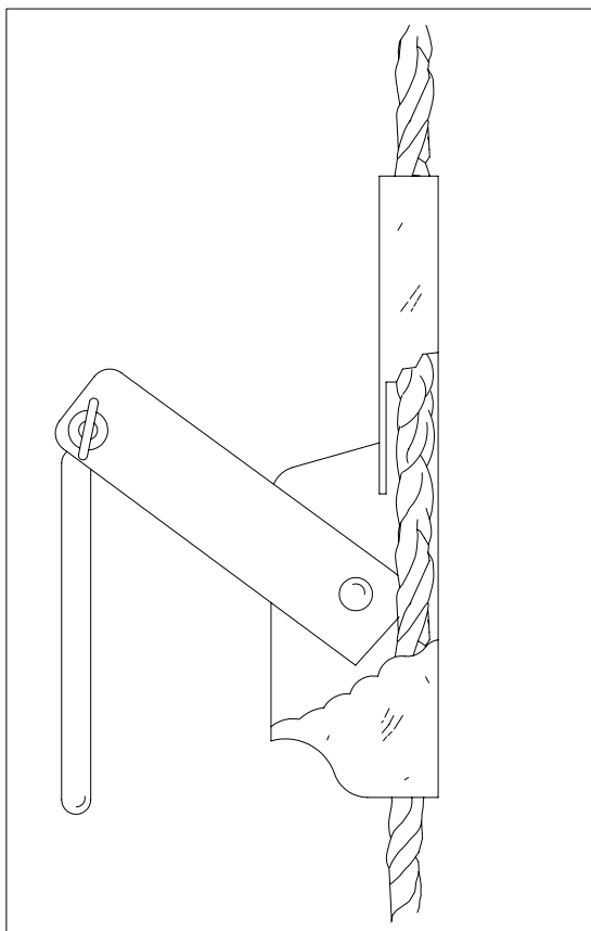
Gancho de seguridad para escaleras
