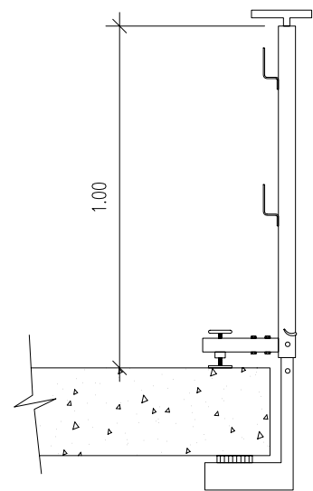
SOPORTE " TIPO - 1 "
