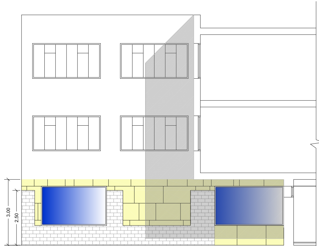
ALZADO ESTE
