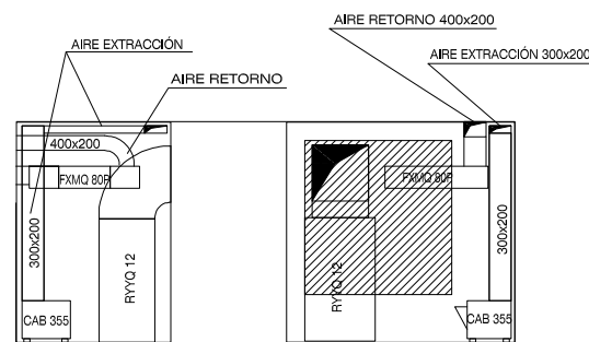
DETALLE INSTALACIÓN CUARTO CLIMA
