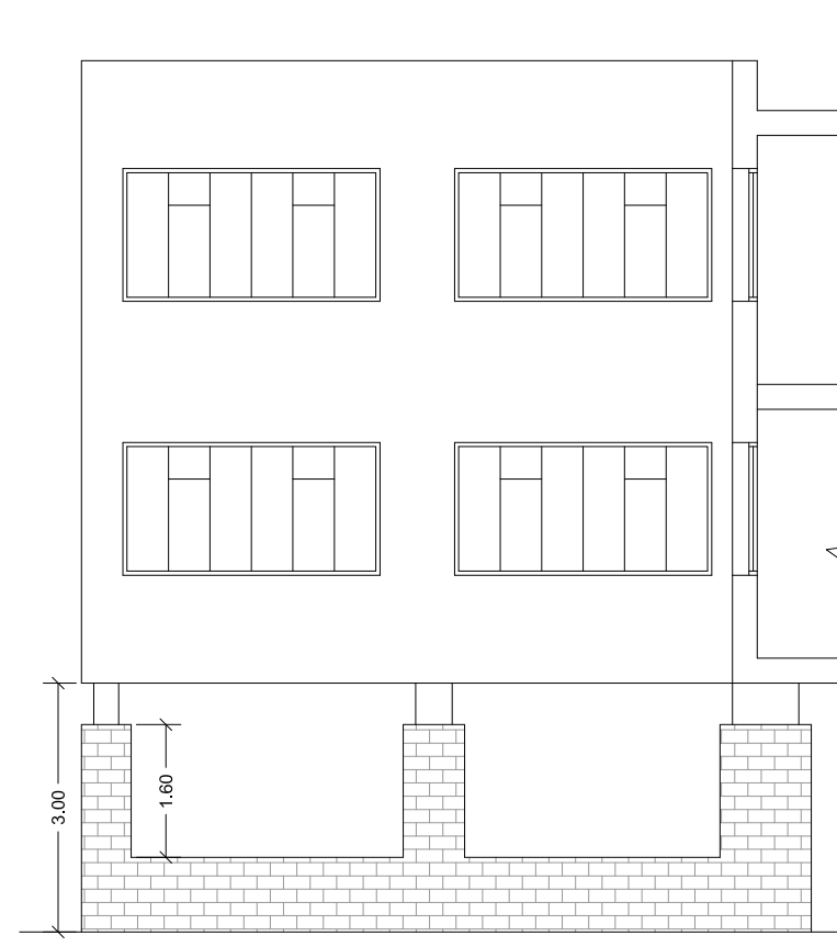
ALZADO ESTE
