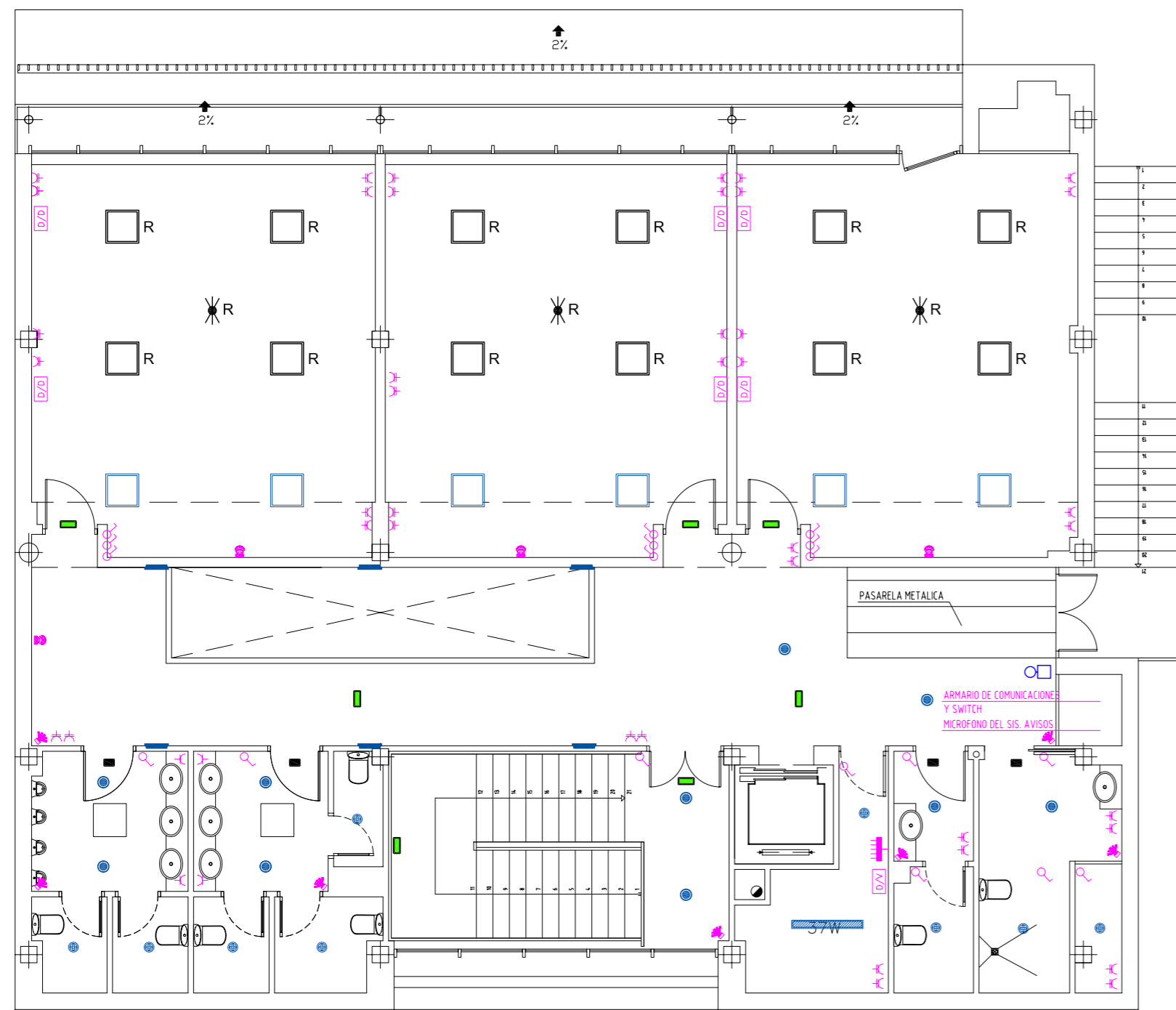
PLANTA PRIMERA
